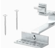
ER-I-SRP-II-TO/02A Verstellbarer Alu-Dachhaken
