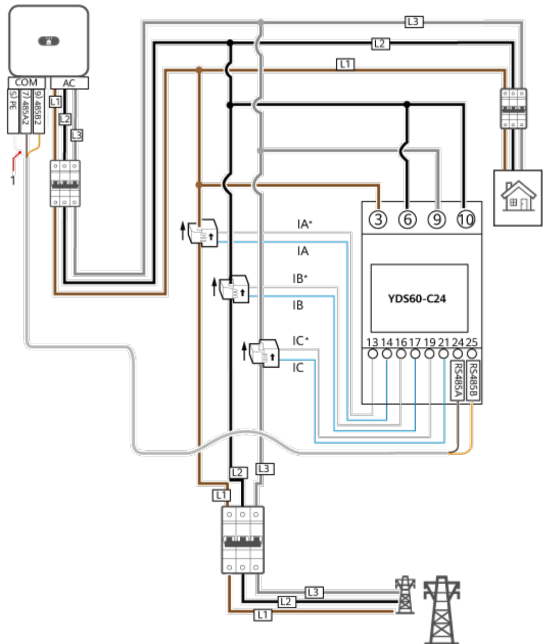
Abbildung 5-24 Dreiphasige, dreiadrige Kabelverbindung mit YDS60-C24 (Smart Dongle-Vernetzung)
