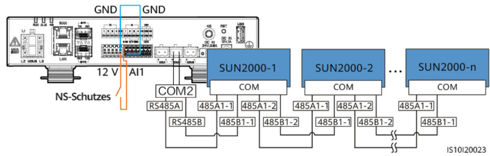
Abbildung 5-42 Anschließen des SmartLoggers an den NS-Schutzschalter
