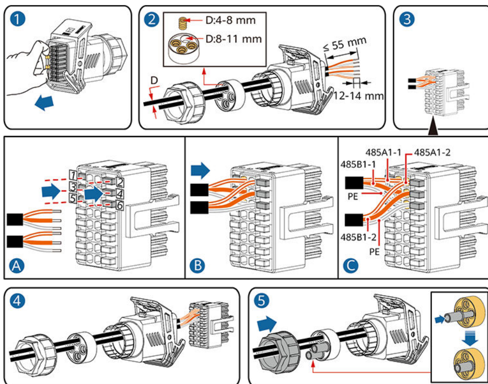
Abbildung 5-21 Kabelmontage
