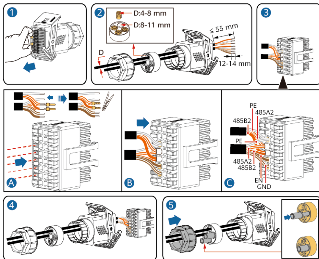
Abbildung 5-32 Kabelmontage
