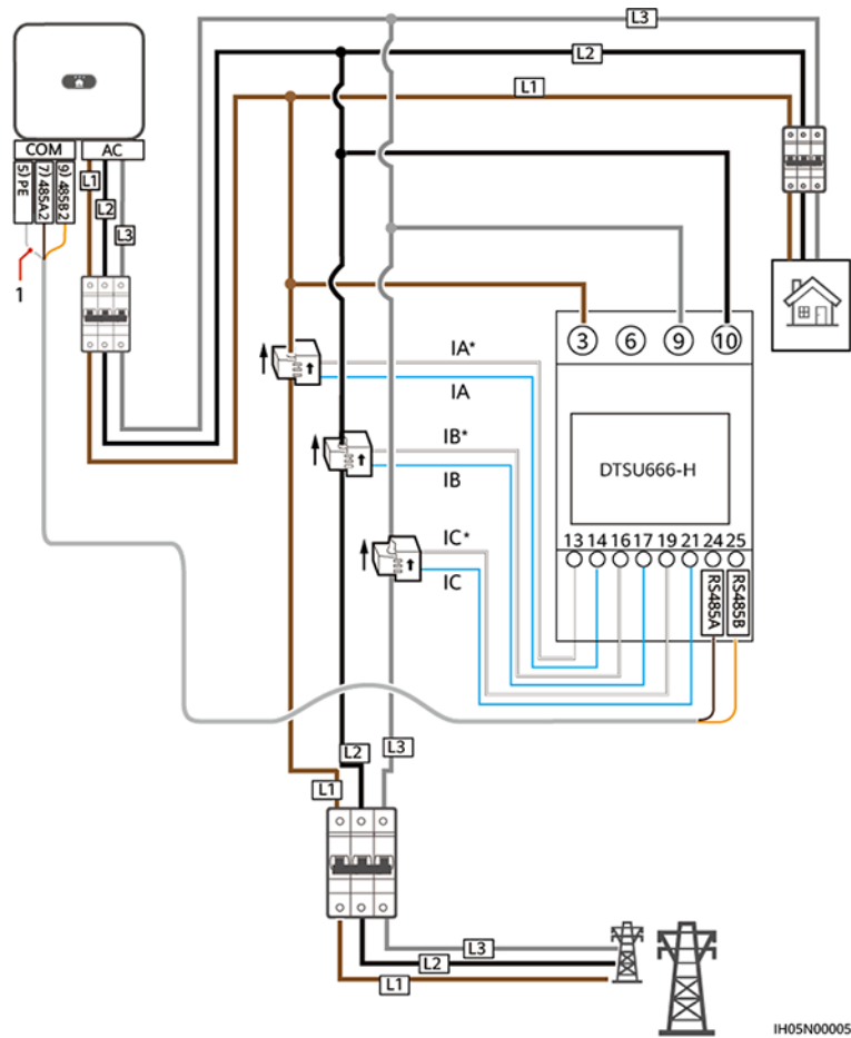
Abbildung 5-23 Dreiphasige, dreidradige Kabelverbindung mit DTSU666-H (Smart Dongle-Vernetzung)
