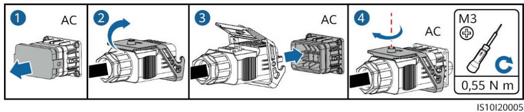
Abbildung 5-9 Sichern des AC-Steckverbinders
