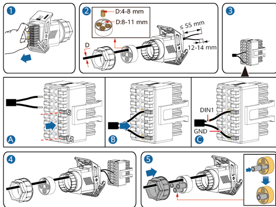
Abbildung 5-37 Kabelmontage
