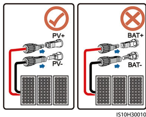
Abbildung 5-12 Korrekte Anschlussklemmen
