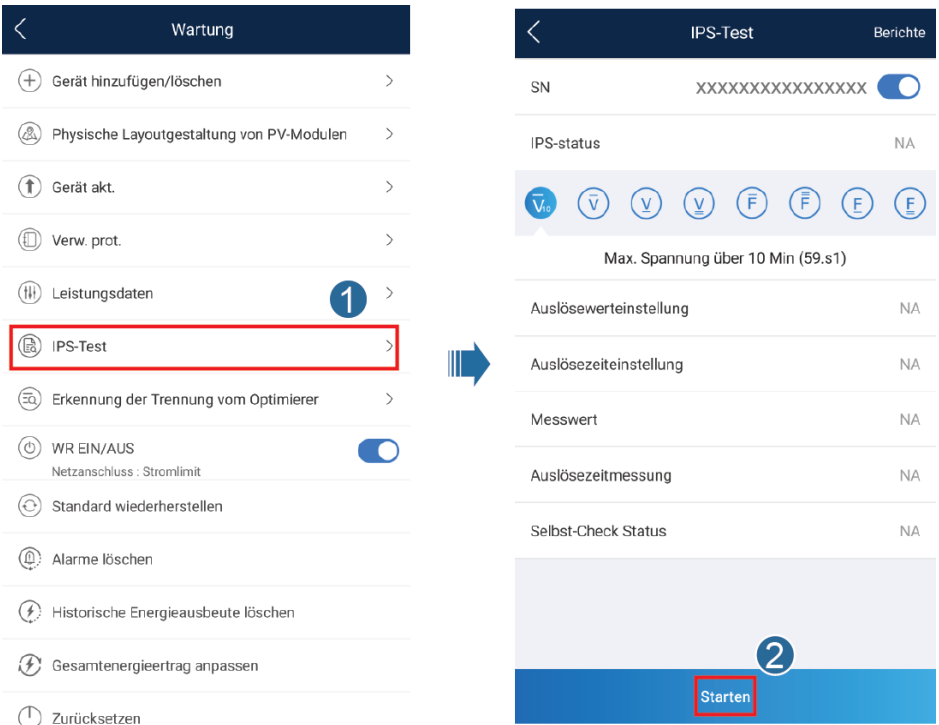
Abbildung 7-18 IPS-Test
