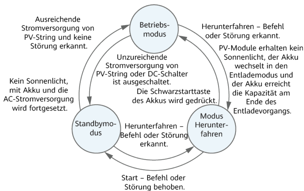
Abbildung 2-7 Arbeitsmodi
