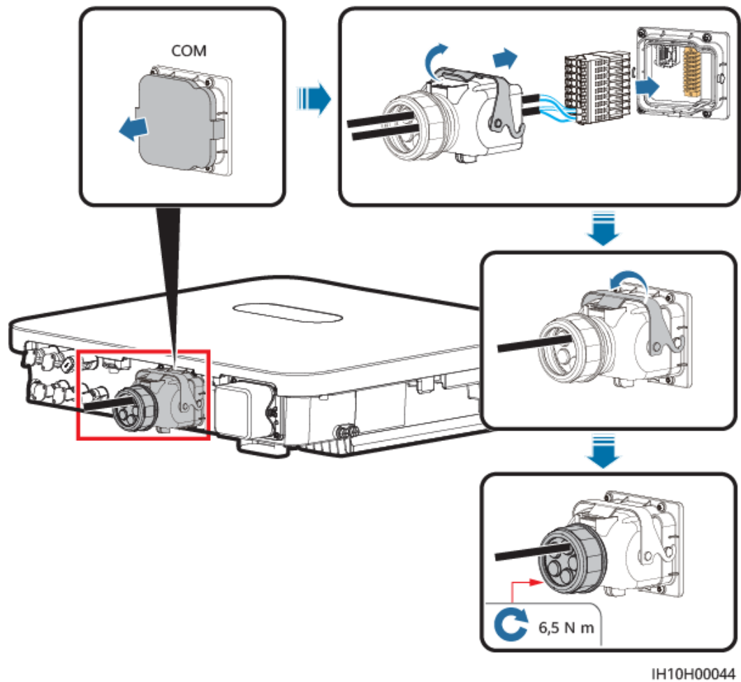
Abbildung 5-38 Sichern des Signalkabelsteckverbinders
