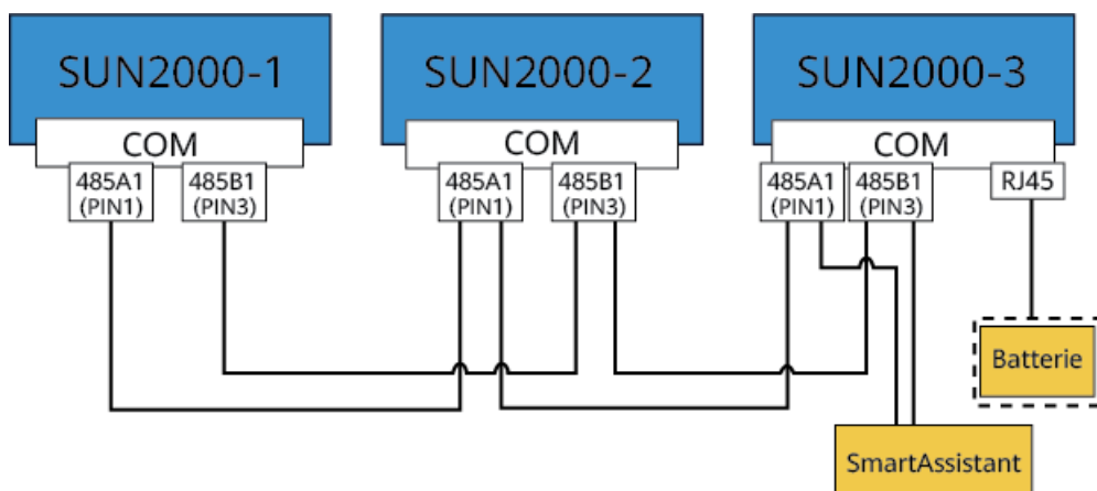
Abbildung 5-16 SmartAssistant-Vernetzung (die Komponente im gestrichelten Kasten ist optional)
