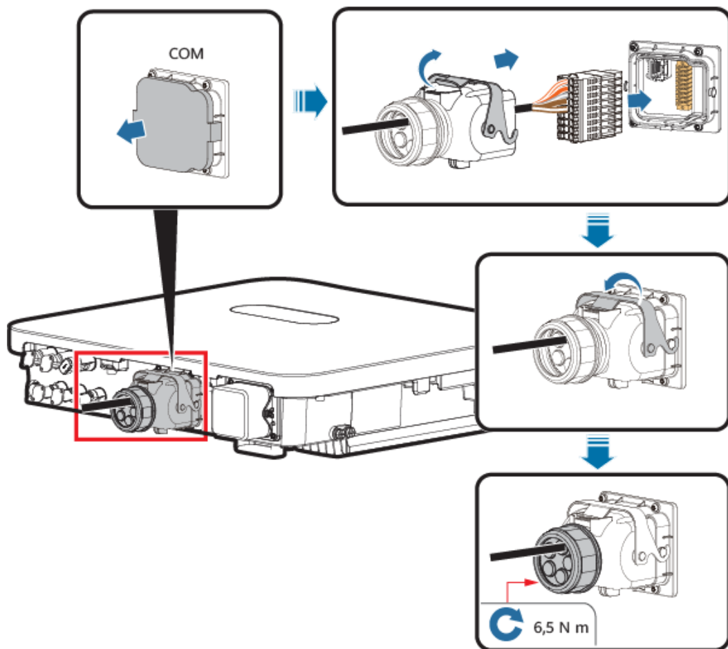
Abbildung 5-29 Sichern des Signalkabelsteckverbinders
