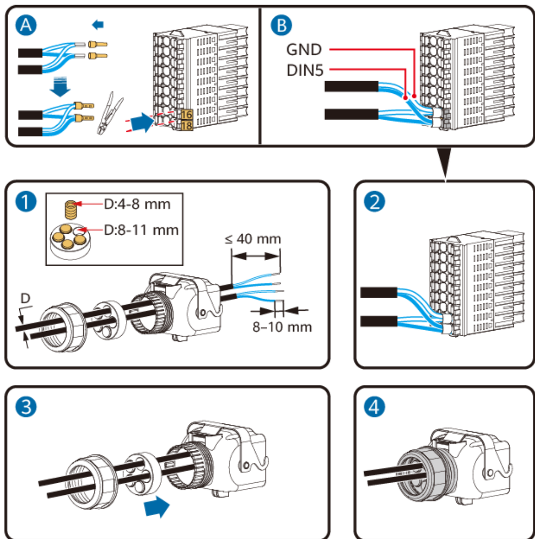
Abbildung 5-31 Kabelmontage
