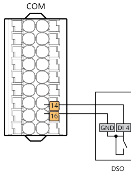
Abbildung 7-12 Kabelverbindungen
