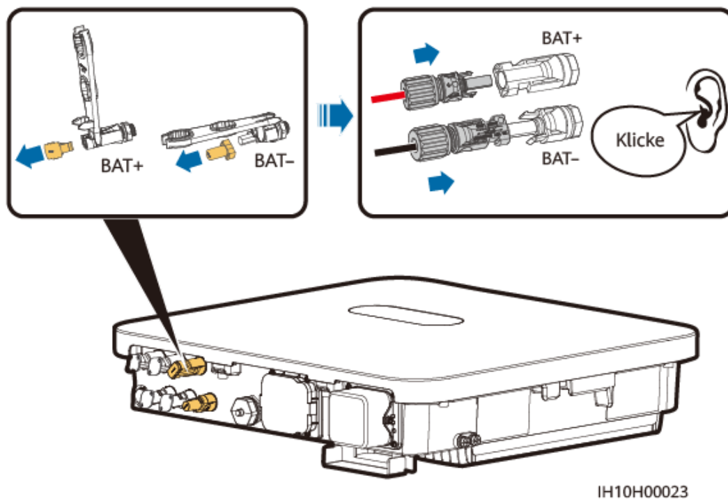
Abbildung 5-12 Anschließen der Batteriekabel
