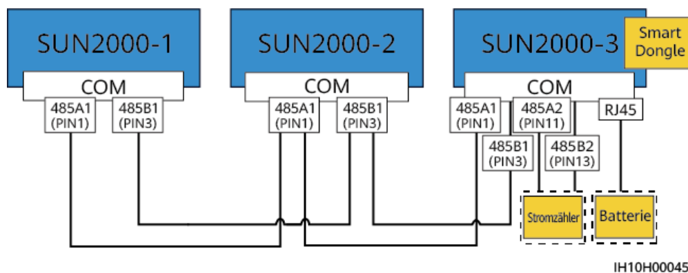
Abbildung 5-15 Smart Dongle-Vernetzung (die Komponente im gestrichelten Kasten ist optional)
