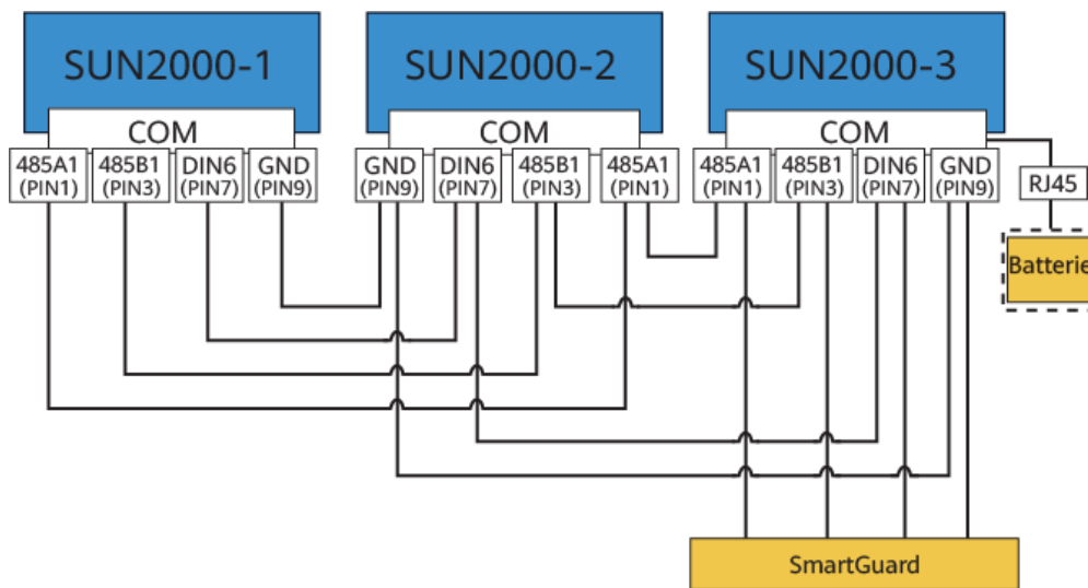
Abbildung 5-17 SmartGuard-Vernetzung (die Komponenten im gestrichelten Kasten sind optional)
