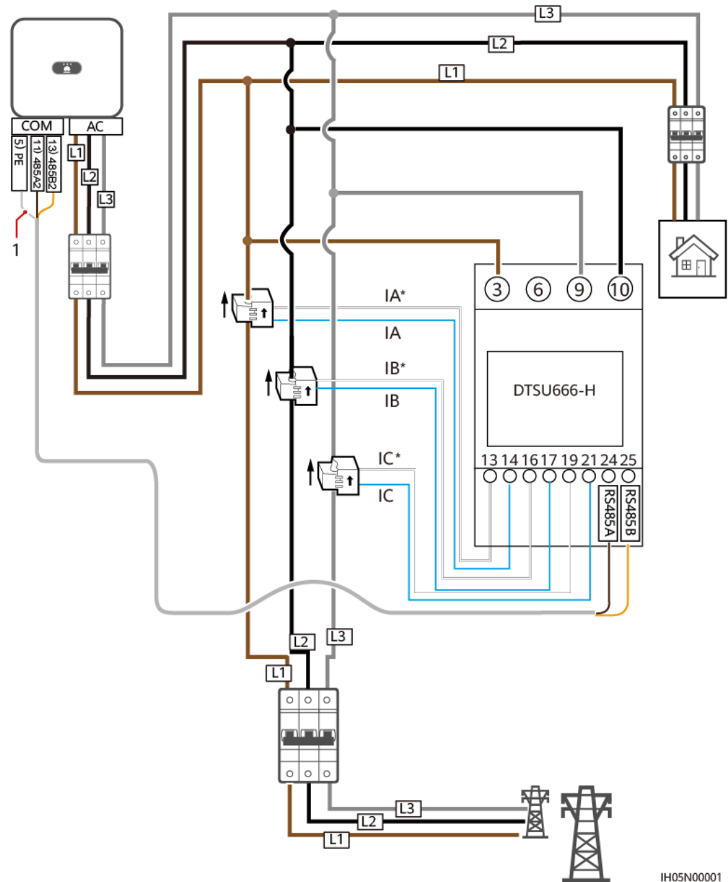
Abbildung 5-21 DTSU666-H dreiphasige dreiadrige Kabelverbindung (Smart Dongle-Vernetzung)
