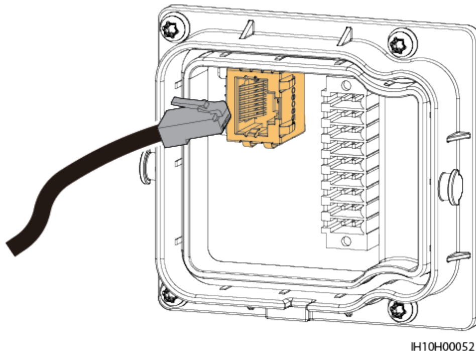
Abbildung 5-40 Kabelmontage
