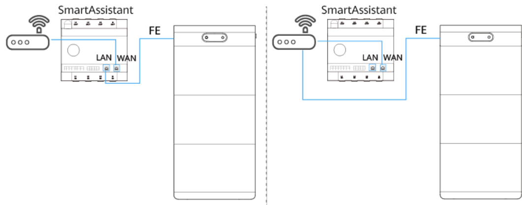
Abbildung 5-8 Netzwerkanschluss mit dem SmartAssistant oder dem Router verbunden
