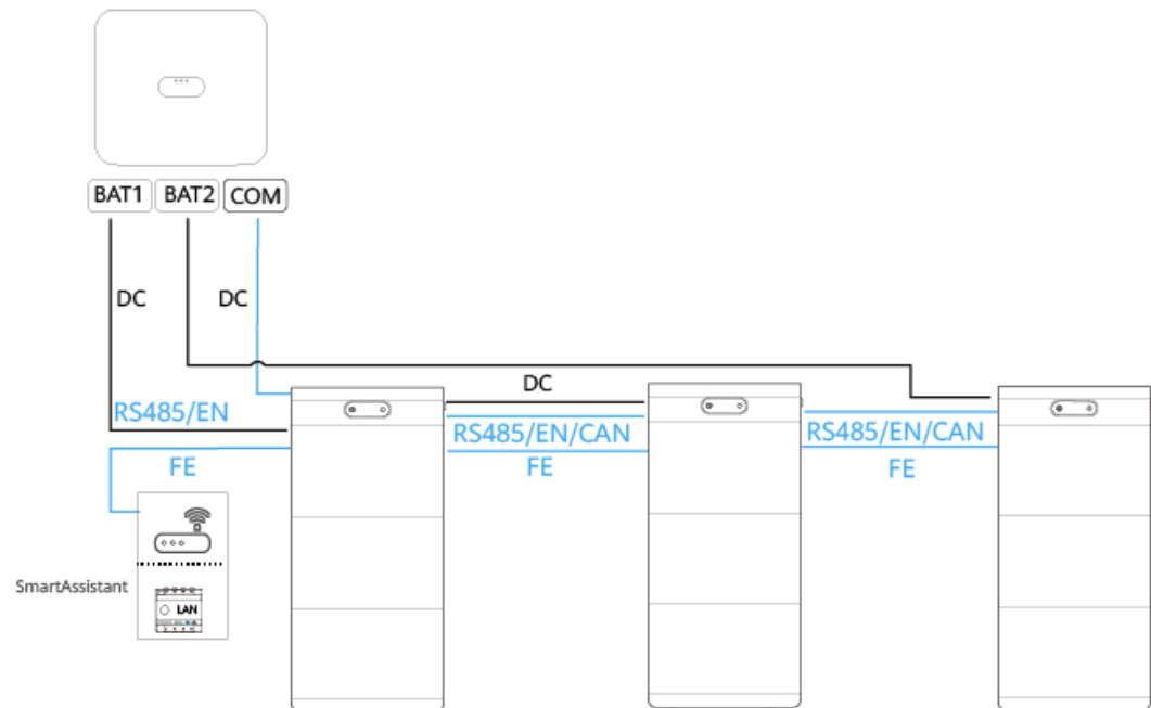
Abbildung 2-12 Anschließen der ESSs an den Wechselrichter (3)
