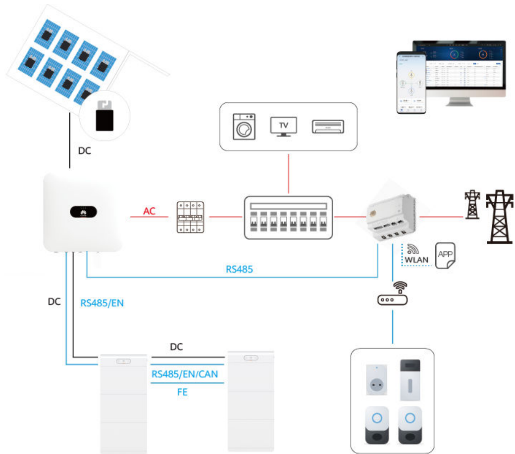
Abbildung 2-9 Netzwerkanschluss mit dem SmartAssistant oder dem Router verbunden
