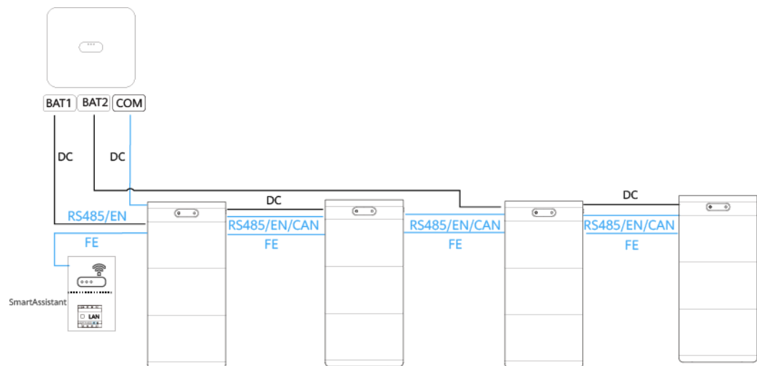
Abbildung 2-13 Anschließen der ESSs an den Wechselrichter (4)
