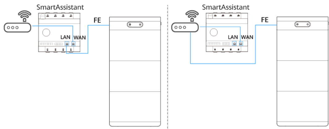
Abbildung 2-9 Netzwerkanschluss mit dem SmartAssistant oder dem Router verbunden
