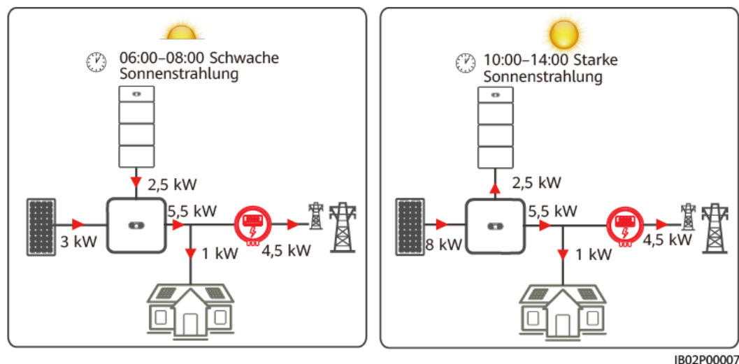
Abbildung 2-15 Komplett ins Netz einspeisen
