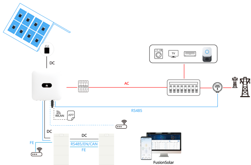
Abbildung 2-7 Netzgekoppeltes Szenario
