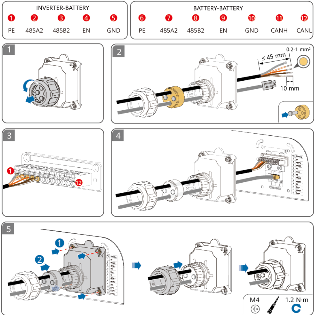
Abbildung 5-7 Signalanschlussverbindungen
