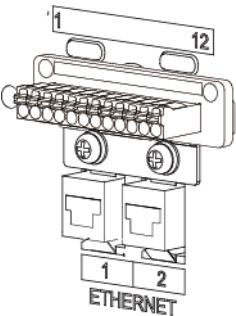
Abbildung 5-5 Signalanschluss
