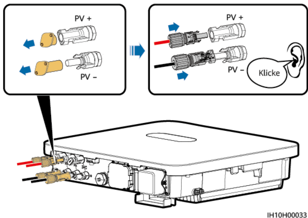
Abbildung 5-10 Anschließen der DC-Eingangsstromkabel
