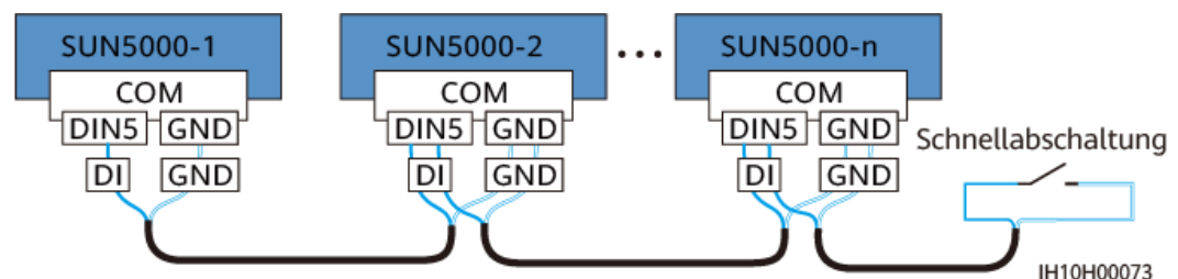
Abbildung 5-30 Anschließen von kaskadierten Wechselrichtern an den Schnellabschaltungsschalter
