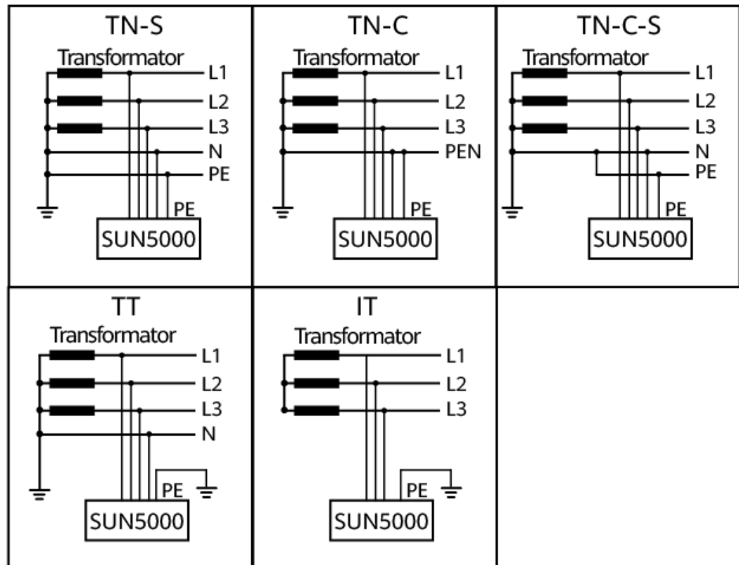
Abbildung 2-7 Erdungssysteme
