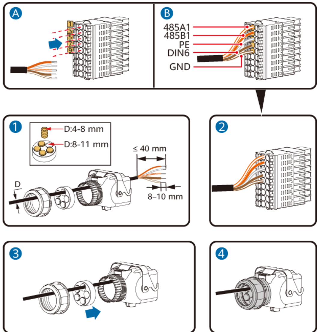
Abbildung 5-28 Kabelmontage
