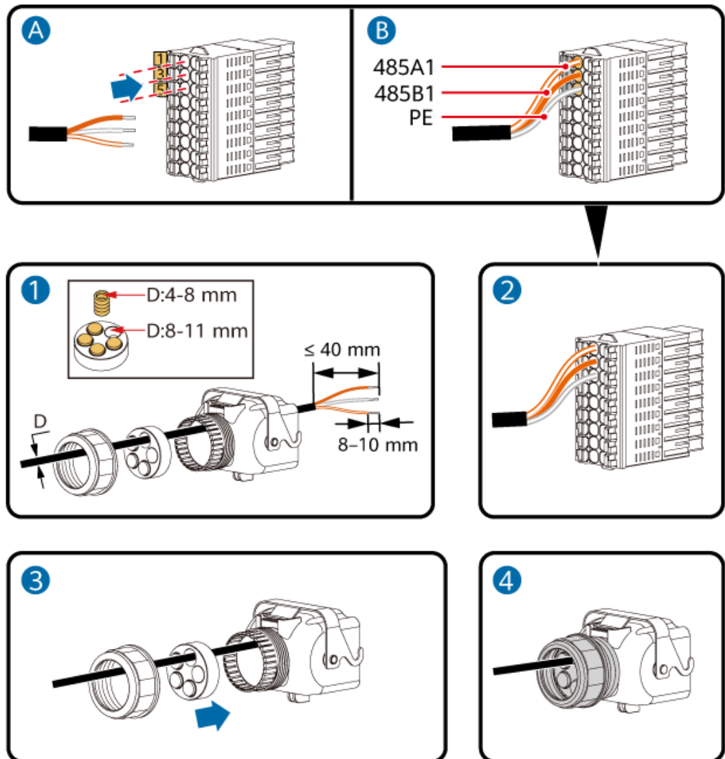
Abbildung 5-26 Kabelmontage
