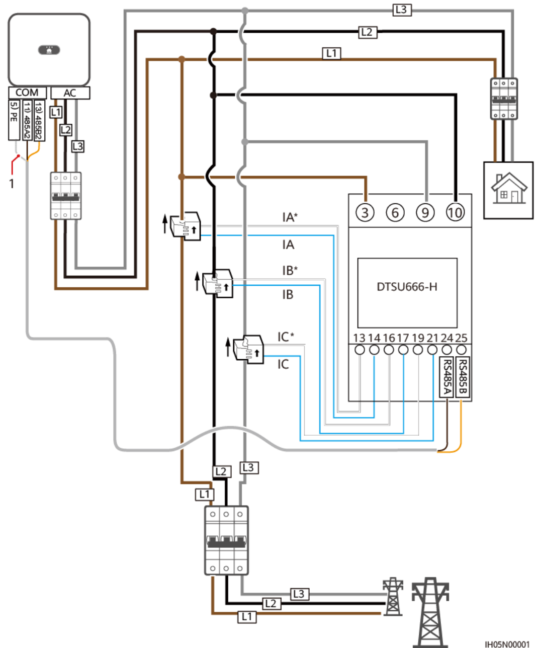
Abbildung 5-21 DTSU666-H dreiphasige dreiadrigte Kabelverbindung (Smart Dongle-Vernetzung)
