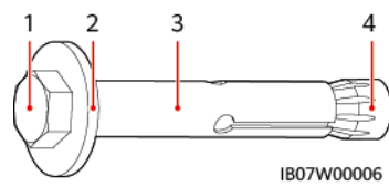
Abbildung 4-7 Struktur der Dehnschraube
