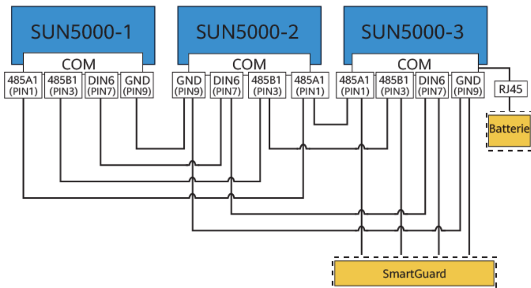
Abbildung 5-17 SmartGuard-Vernetzung (gestrichelte Kästchen stehen für optionale Komponenten.)
