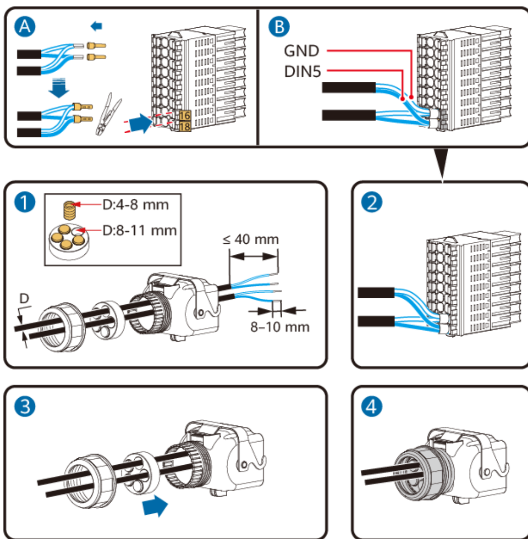
Abbildung 5-31 Kabelmontage
