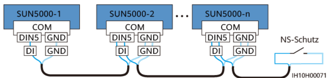
Abbildung 5-36 Anschließen von kaskadierten Wechselrichtern an den NS-Schutzschalter
