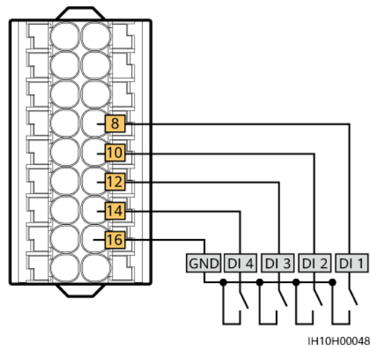
Abbildung 5-33 Kabelverbindung
