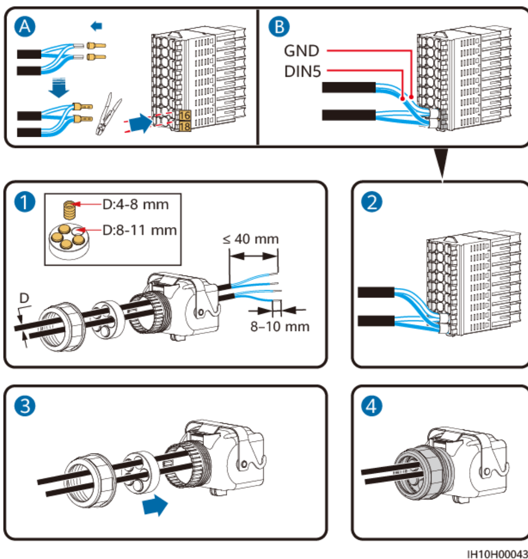
Abbildung 5-37 Installieren von Kabeln
