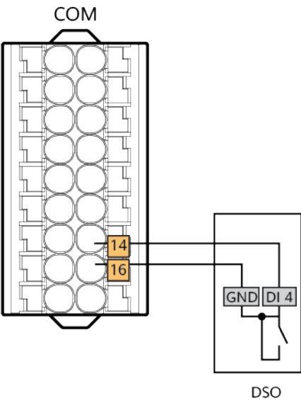
Abbildung 7-6 Kabelverbindungen
