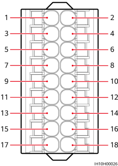
Abbildung 5-13 COM: 18-polige Klemme
