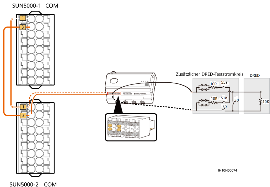
Abbildung 7-11 Verdrahtungsplan für die DRM-Funktion (SmartAssistant-Vernetzung)
