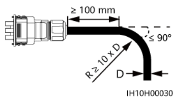
Abbildung 5-6 Verkabelungsanforderungen
