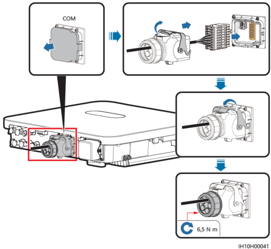
Abbildung 5-35 Sichern des Signalkabelsteckverbinders
