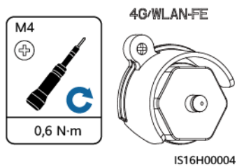
Abbildung 5-44 Installation der Anti-Diebstahl-Komponenten für den Smart Dongle
