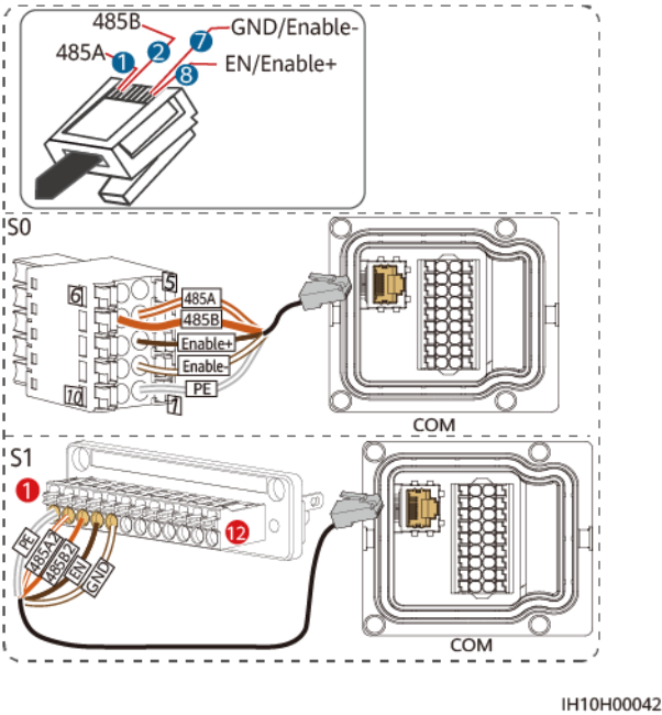
Abbildung 5-39 Kabelverbindung
