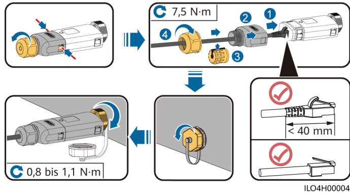
Abbildung 5-41 Installieren von WLAN-FE-Smart Dongle (FE-Kommunikation)
