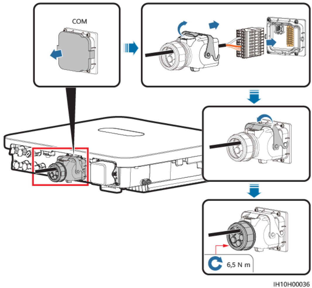
Abbildung 5-25 Sichern des Signalkabelsteckverbinders
