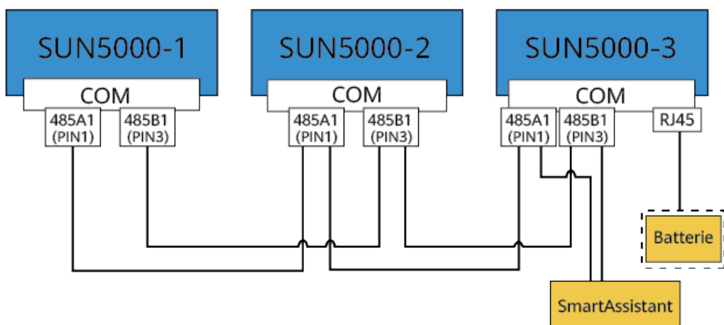
Abbildung 5-16 SmartAssistant-Vernetzung (gestrichelte Kästchen stehen für optionale Komponenten.)
