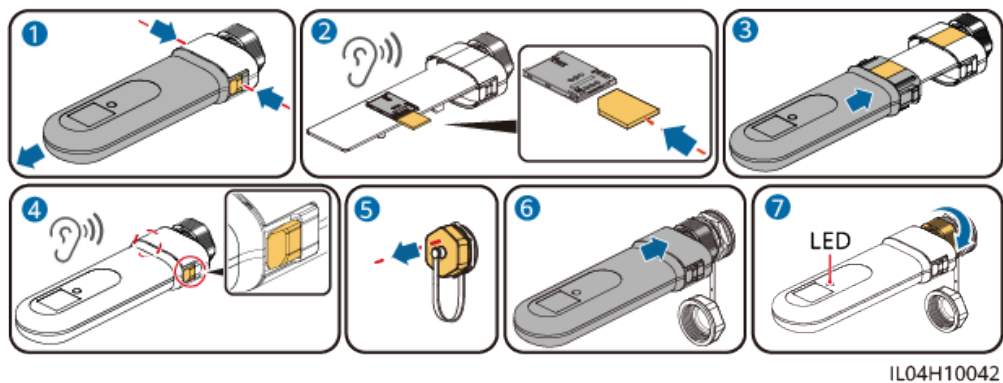
Abbildung 5-43 Installieren von 4G Smart Dongle (SDongleB-06)
