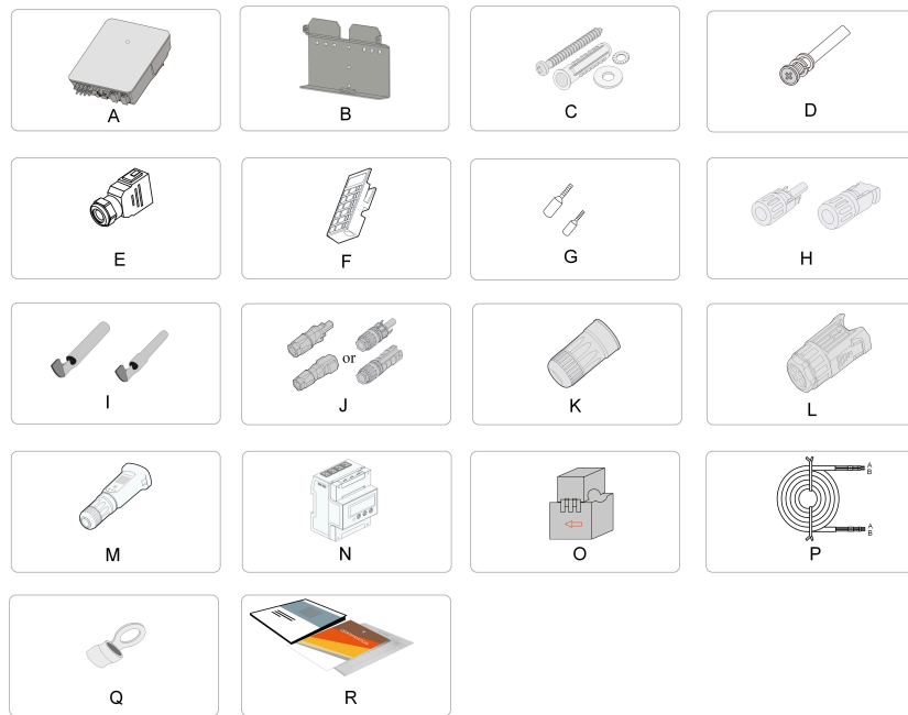
Abbildung 4-1 Lieferumfang
