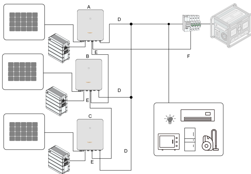
Abbildung 2-5 Netzunabhängig zentralisiert mit Last
