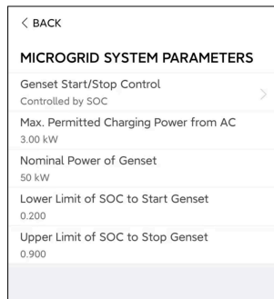
Abbildung 8-36 MicroGrid System Parameters
