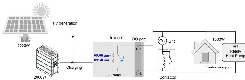
Abbildung 8-33 DO-Betrieb im intelligenten Modus
