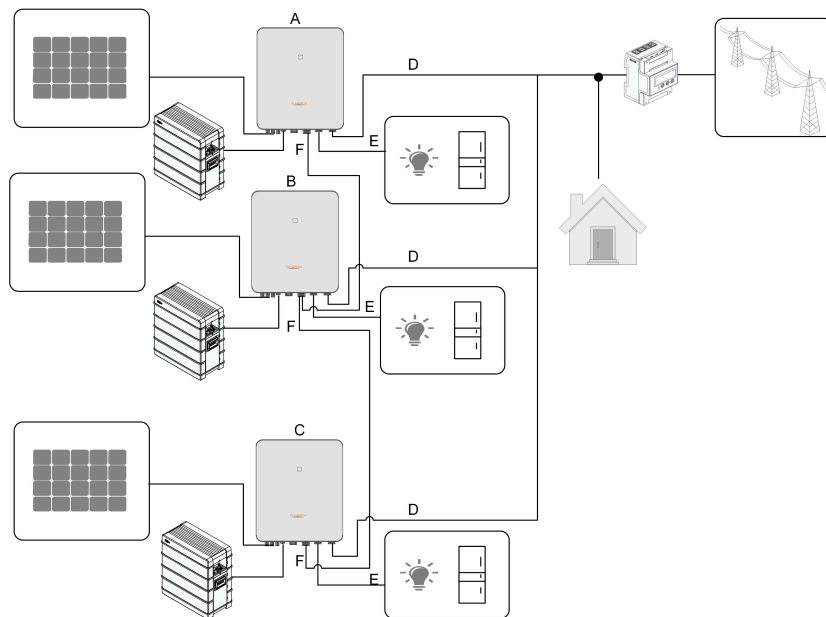
Abbildung 2-4 Paralleles PV ESS
