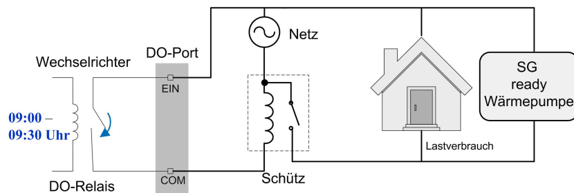
Abbildung 8-31 DO-Schalter steuert zeitlich ein Relais für zuschaltbare Verbraucher an
