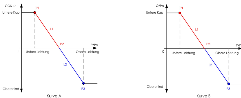
Abbildung 8-4 Q(P)-Kurve
