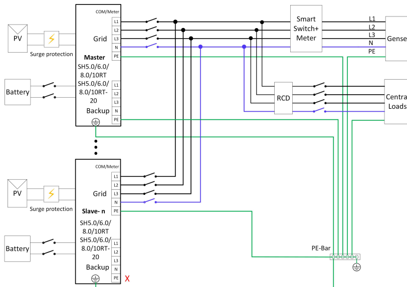
Abbildung 2-7 Schaltplan für andere Regionen *
