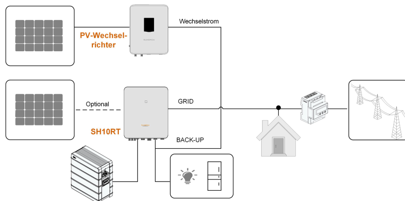
Abbildung 2-10 Backup-Anschluss zur Nachrüstung der bestehenden PV-Anlage
