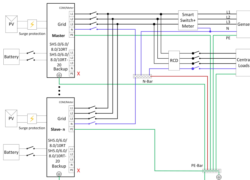
Abbildung 2-6 Verdrahtungsplan für Australien und Neuseeland
