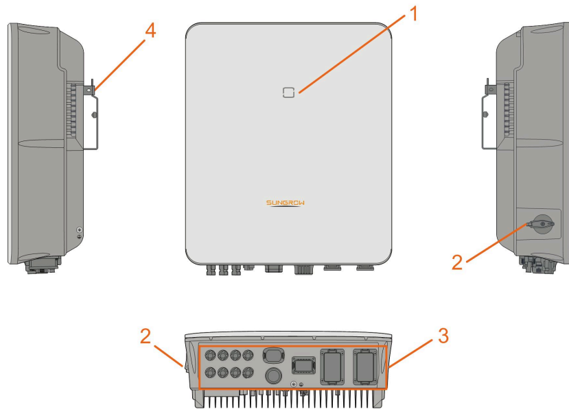
Abbildung 2-1 Geräteansicht
