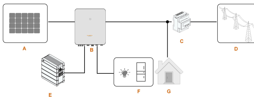
Abbildung 2-3 Das PV-Energiespeichersystem System (PV ESS)
