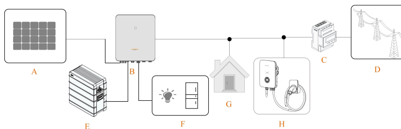
图 8: PV-Speicher und EV-Ladesystem
