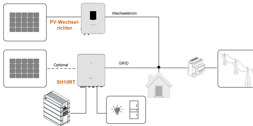
Abbildung 2-9 Netzgekoppelter Anschluss zur Nachrüstung der bestehenden PV-Anlage
