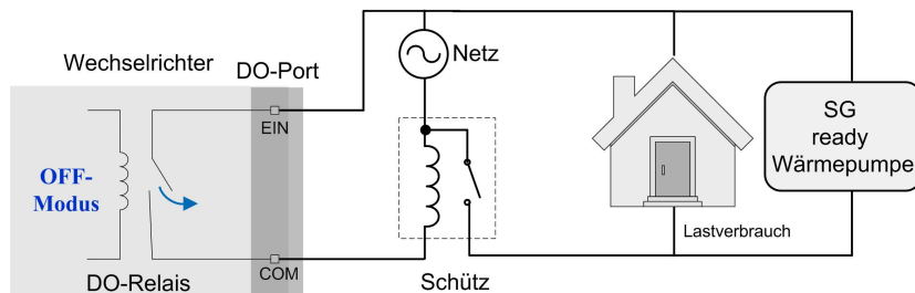
Abbildung 8-32 DO-Betrieb im Sofortmodus
