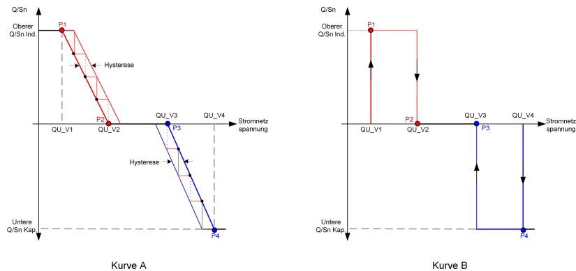
Abbildung 8-5 Q(U)-Kurve
